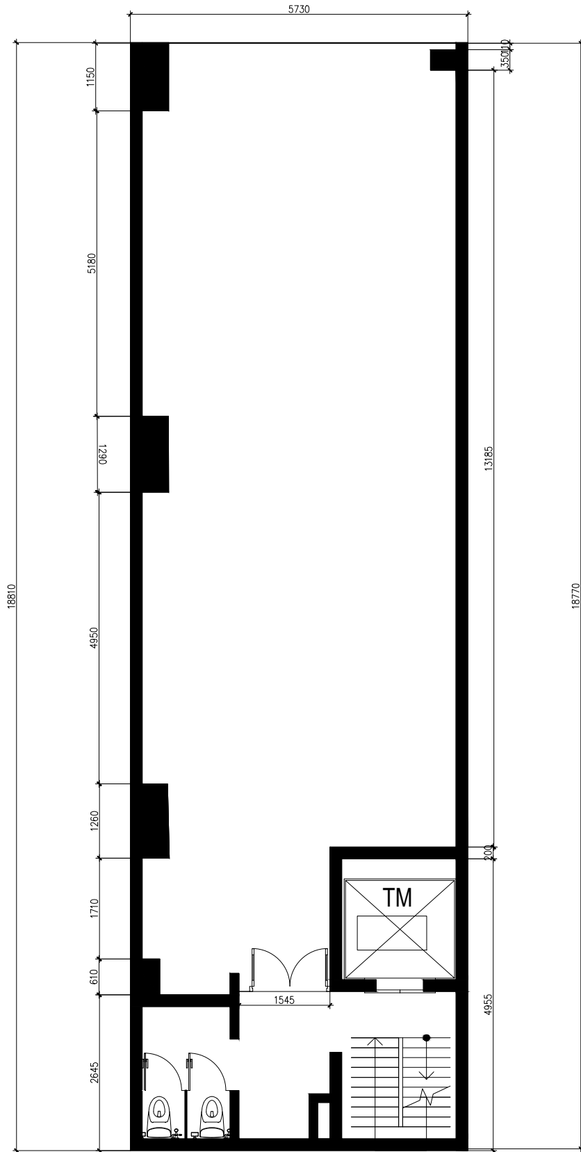
MẶT BẰNG ĐIỂN HÌNH TẦNG 2-6 78 M2
