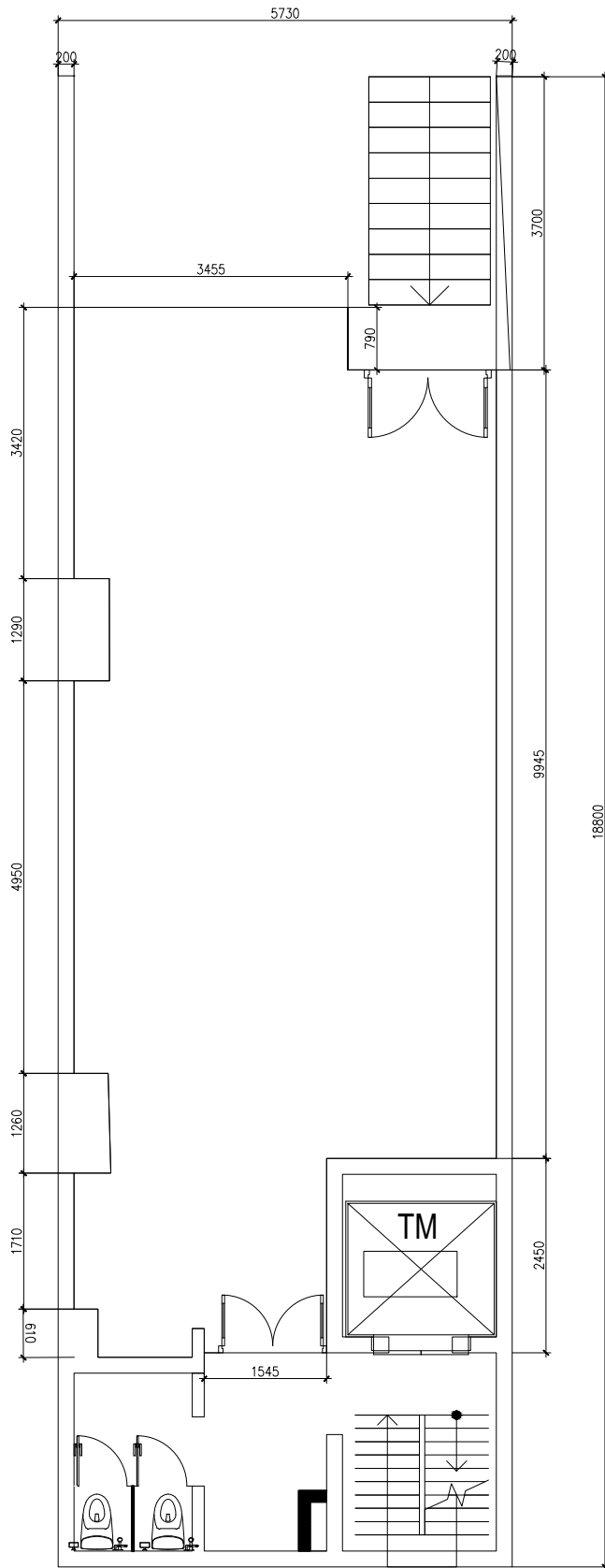
MẶT BẰNG ĐIỂN HÌNH TẦNG 1 62 M2
